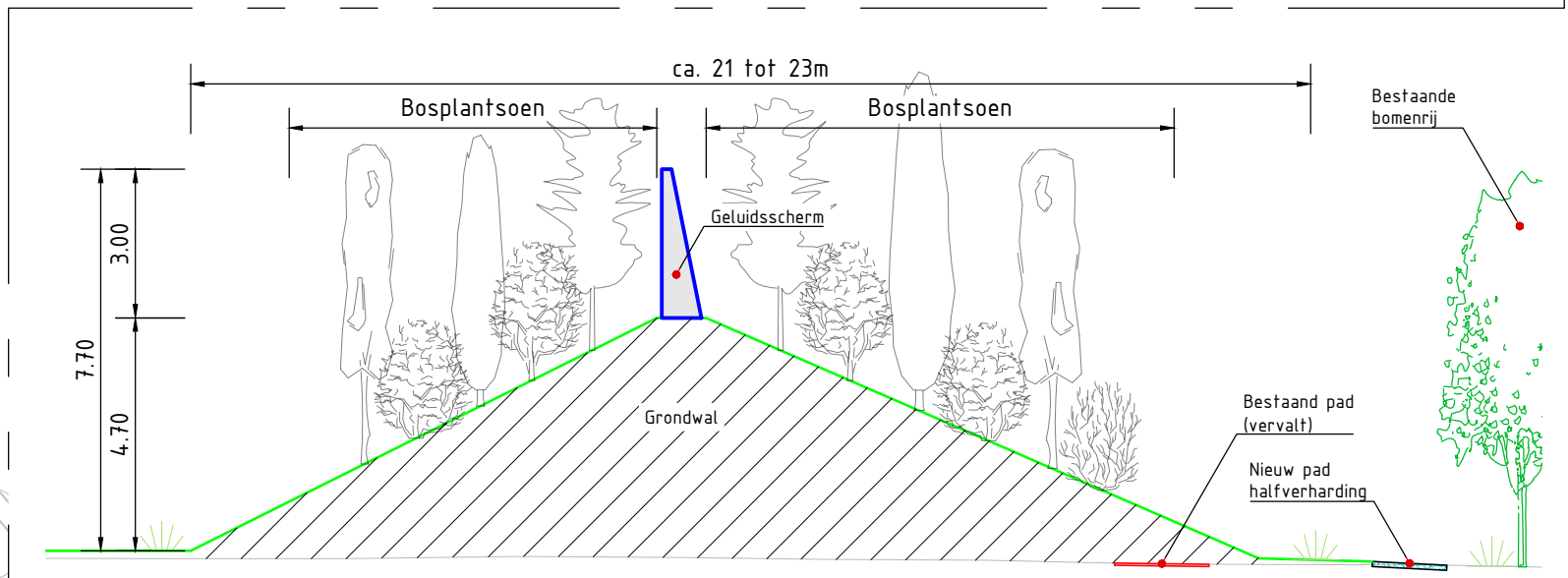
Principe profiel
